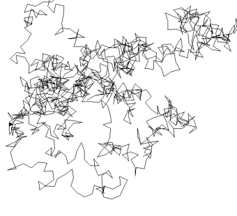
Trajectoire simulée d'une molécule après 1000 collisions
