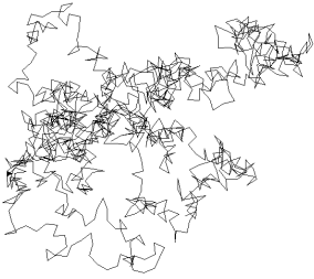
Trajectoire simulée d'une molécule après 1000 collisions
