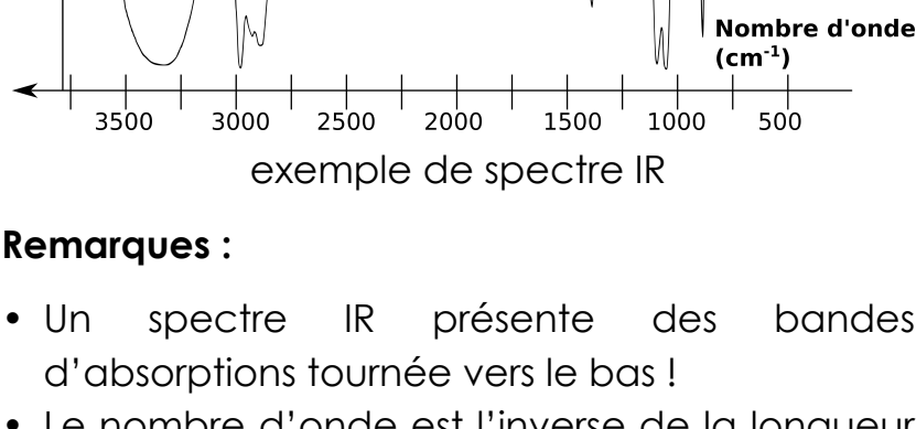
exemple de spectre IR
