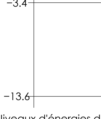
Fig. 2. – Niveaux d'énergies de l'atome d'hydrogène
