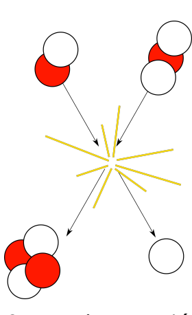
Fig. 2. – Fusion nucléaire
