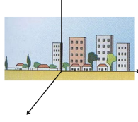
Fig. 1. – Référentiel terrestre Fig. 2. – Référentiel Géocentrique et Héliocentrique
