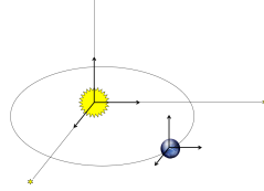
Fig. 1. – Référentiel terrestre Fig. 2. – Référentiel Géocentrique et Héliocentrique
