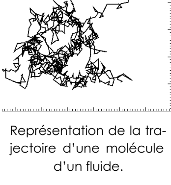
Représentation de la trajectoire d'une molécule d'un fluide.
