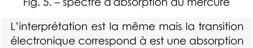
Fig. 5. – spectre d'absorption du mercure
