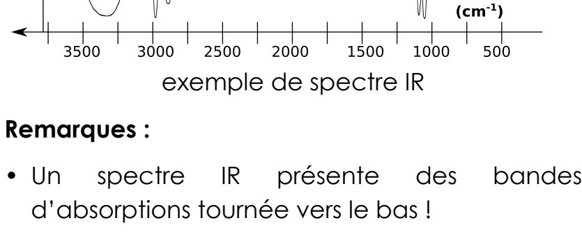
exemple de spectre IR
