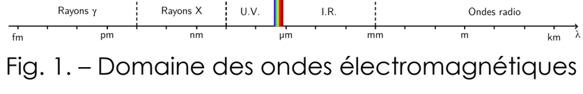
Fig. 1. – Domaine des ondes électromagnétiques
