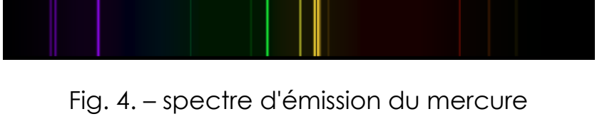
Fig. 4. – spectre d'émission du mercure
