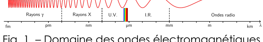
Fig. 1. – Domaine des ondes électromagnétiques
