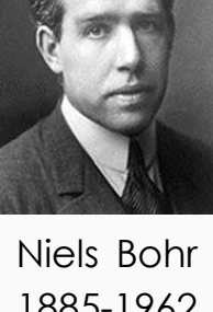
Niels Bohr
