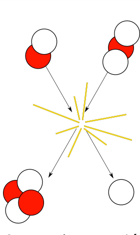
Fig. 2. – Fusion nucléaire
