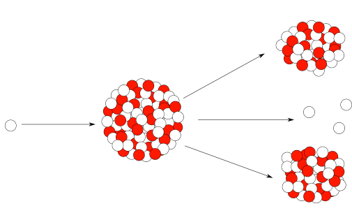
Fig. 3. – Fission nucléaire
