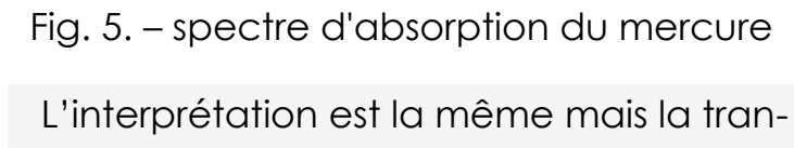
Fig. 5. – spectre d'absorption du mercure
