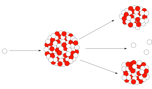
Fig. 3. – Fission nucléaire
