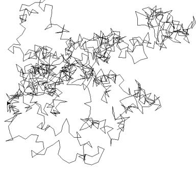
Trajectoire simulée d'une molécule après 1000 collisions
