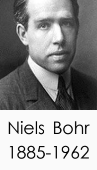
Niels Bohr 1885-1962
