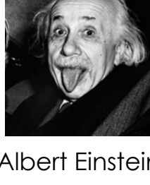
Albert Einstein 1879-1955
