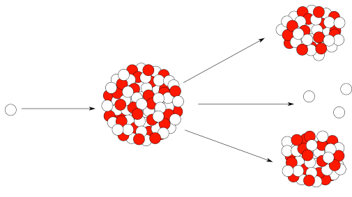
Fig. 3. – Fission nucléaire
