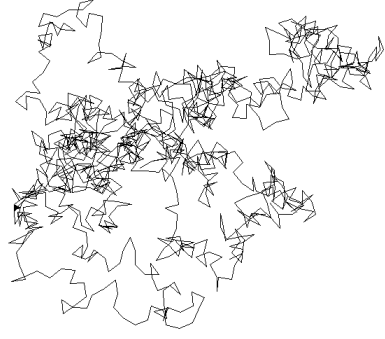
Trajectoire simulée d'une molécule après 1000 collisions
