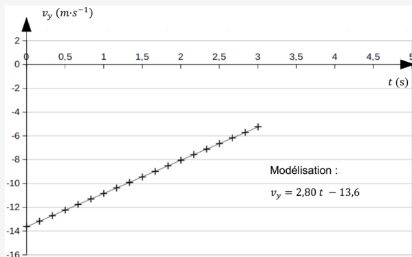
Fig. 1. – Évolution de la coordonnée verticale v_y du vecteur vitesse du point M en fonction du temps.
