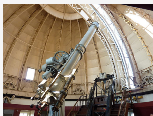
Grande lunette astronomique de l'observatoire de Strasbourg
