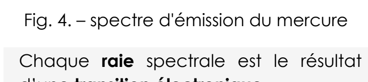
Fig. 4. – spectre d'émission du mercure
