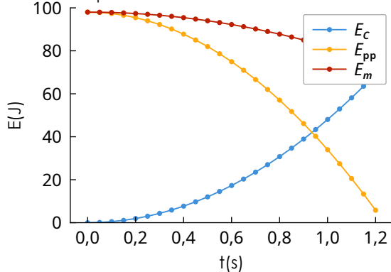
Diminution de l'énergie mécanique pour une chute avec frottements
