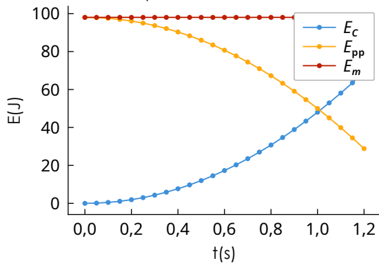
Conservation de l'énergie mécanique pour une chute libre
