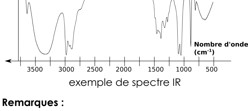
exemple de spectre IR
