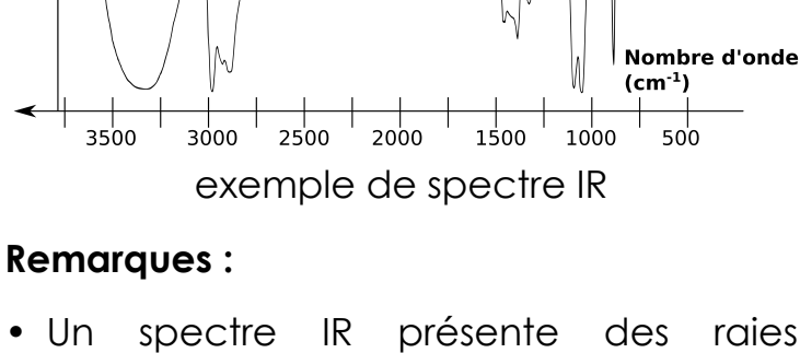
exemple de spectre IR
