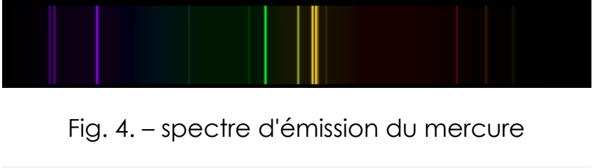
Fig. 4. – spectre d'émission du mercure
