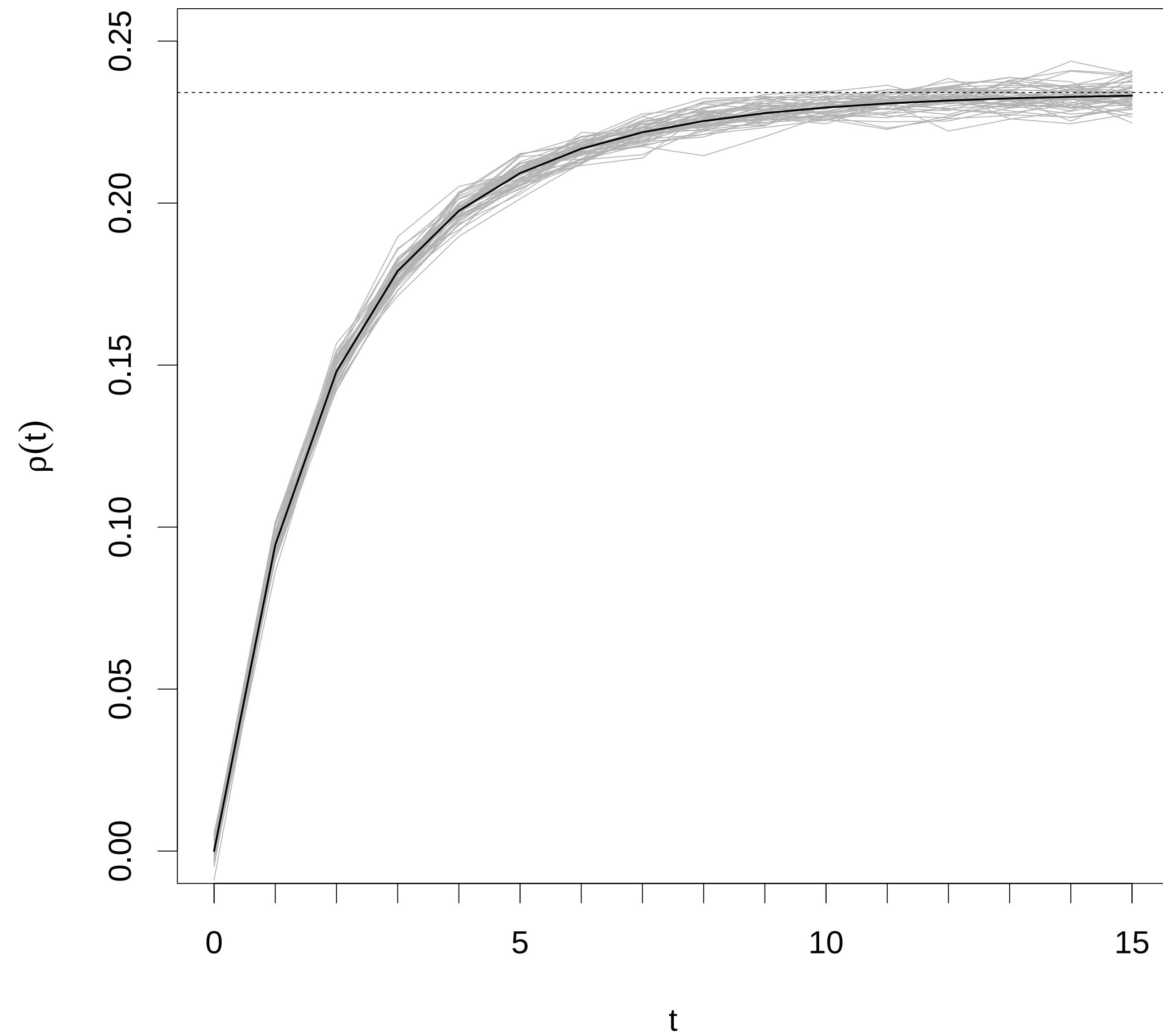
population size 100,000
