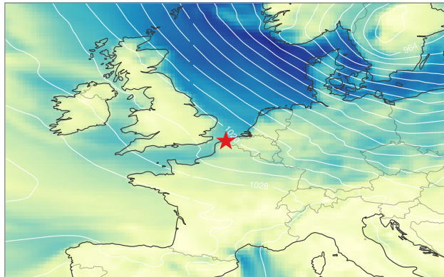
b Xavier (Dec 2013), Dunkerque GEFS +45 h, valid 2013-12-05 21 UTC
