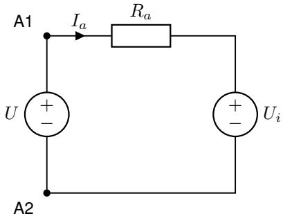
obvod kotvy
