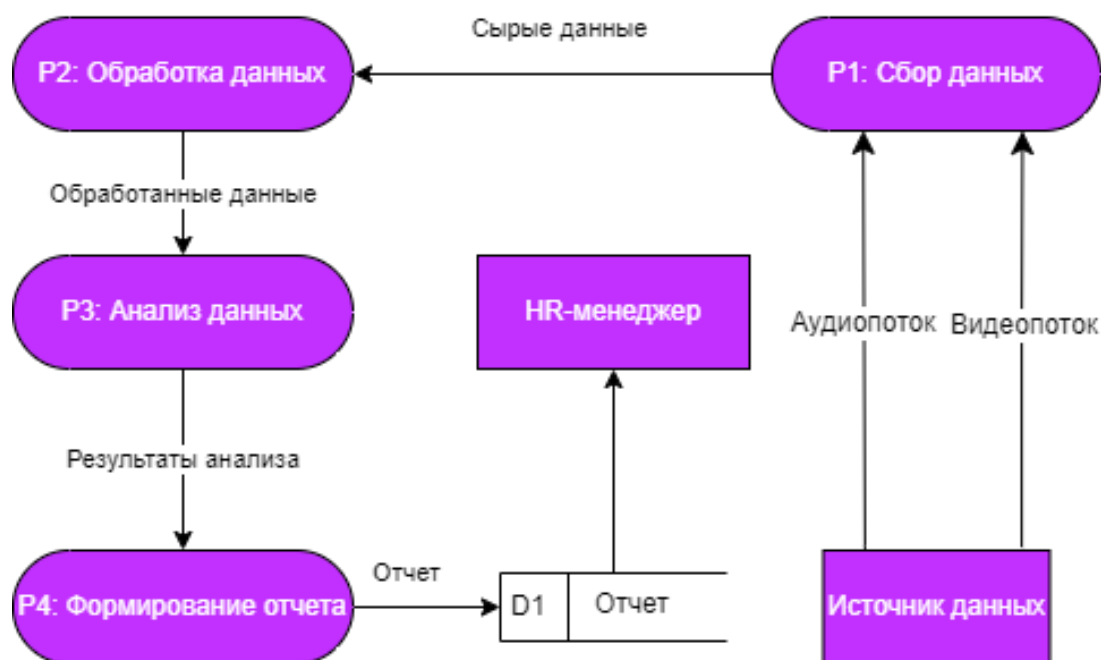
Рисунок 4. DFD диаграмма системы
