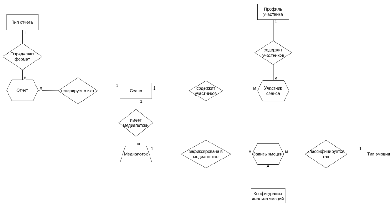
Рисунок 12. Логическая модель базы данных
