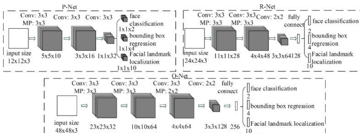
Рисунок 10 – Архитектура MTCNN
