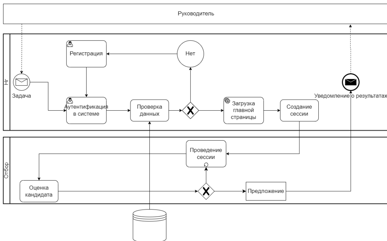
Рисунок 1 – BPMN-диаграмма существующего бизнес-процесса оценки кандидатов до внедрения системы распознавания эмоций
