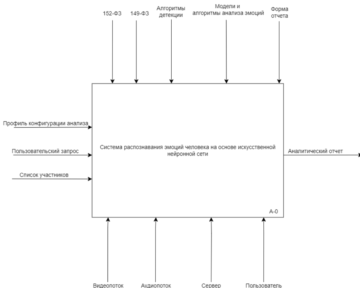
Рисунок 3 – IDEF0-диаграмма системы
