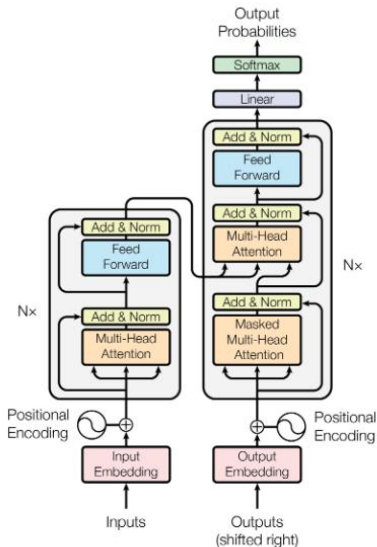
Рисунок 14 – Архитектура Transformer
