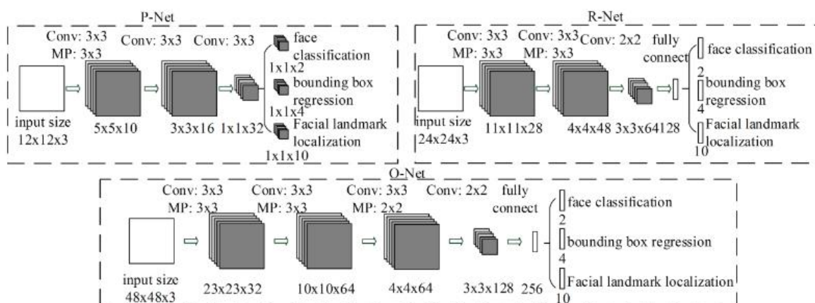
Рисунок 10 – Архитектура MTCNN
