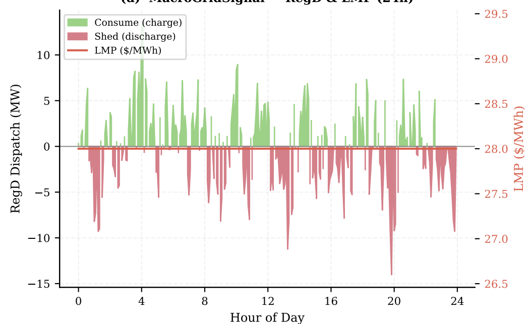
(d) MacroGridSignal — RegD & LMP (24h)
