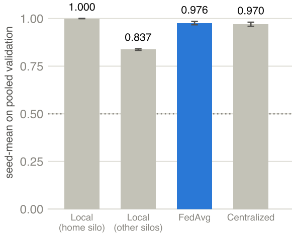
Subtype (AUROC)
