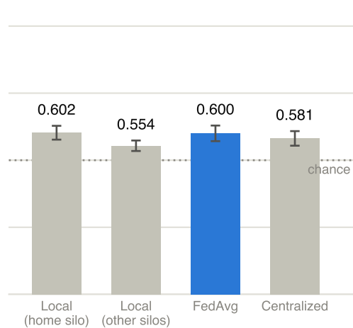
OS (C-index)
