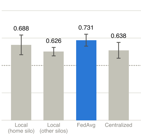
EGFR (AUROC)
