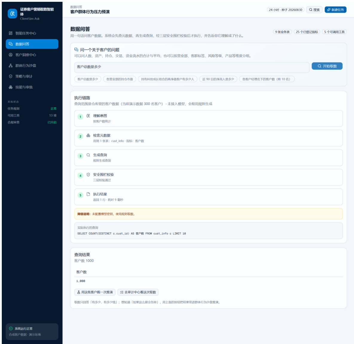
图 4 数据问答：五步执行链路、实际执行的查询与安全围栏校验结果
