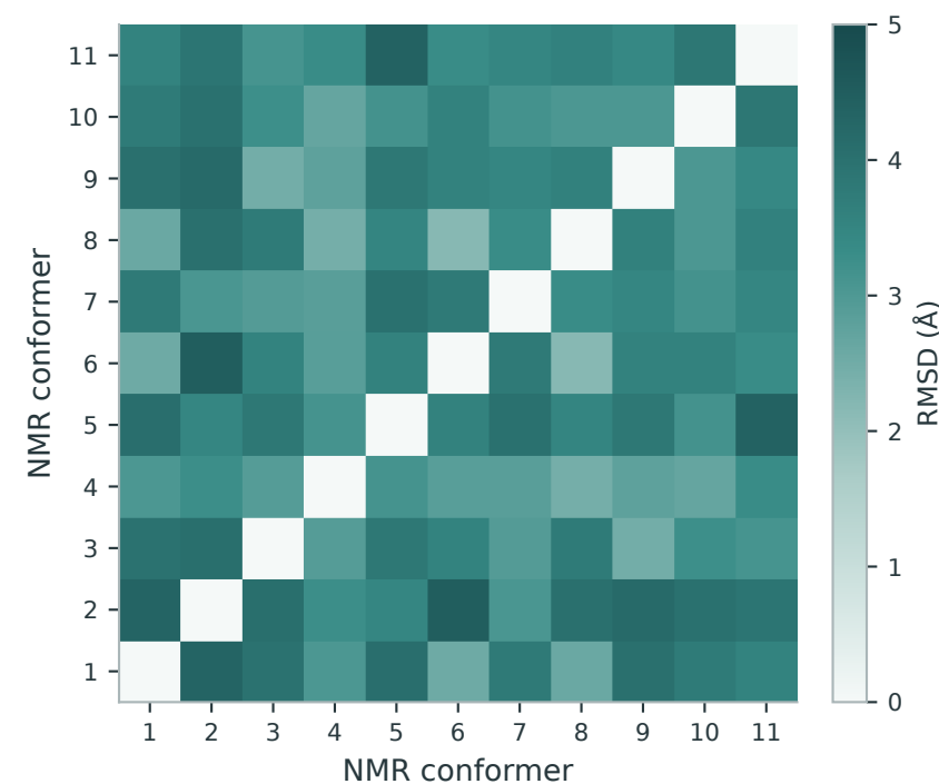
b Pairwise best-fit Cα RMSD (1-57)
