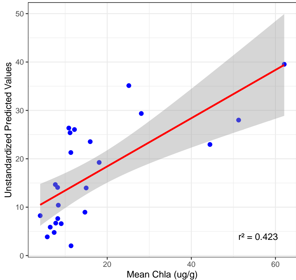
Actual vs Predicted Values for Chla
