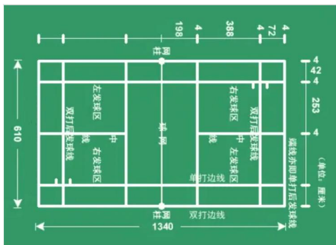
图 1-4 羽毛球双打地胶场地尺寸
