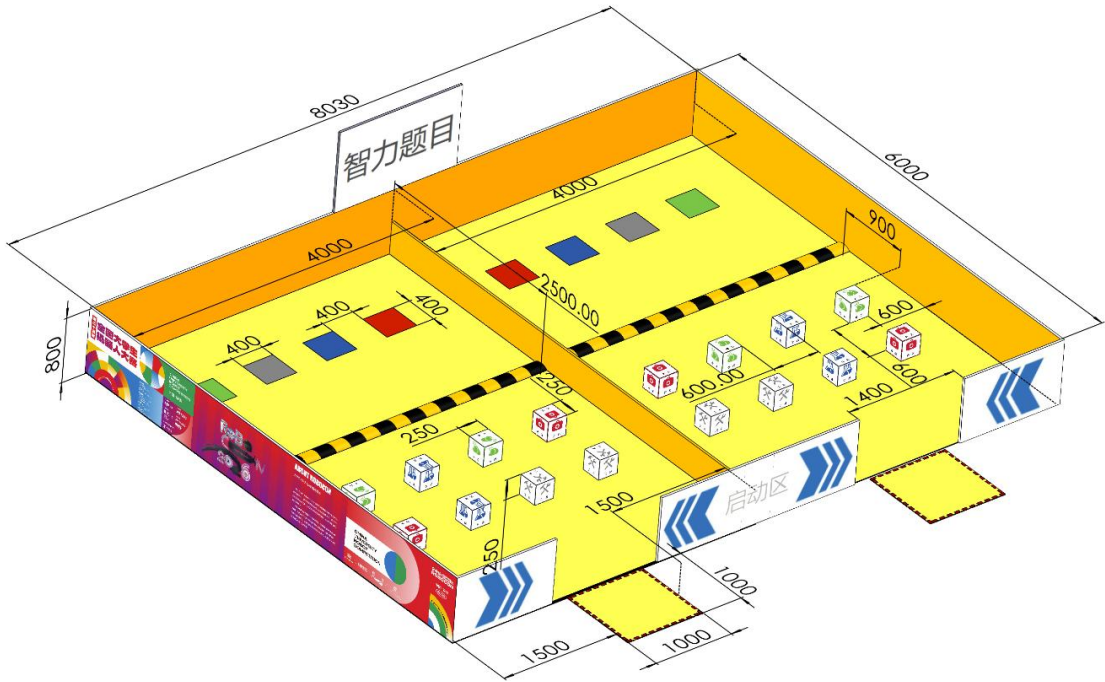
图 1-3 任务赛场地透视图
