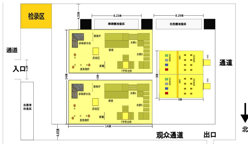
图 2-4 国际交流中心仿生足式机器人比赛场地
