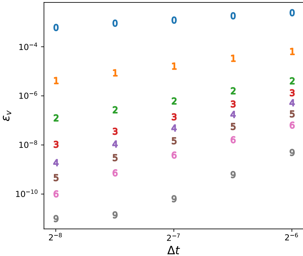
Vortex TG -- SDC(3,k) convergence
