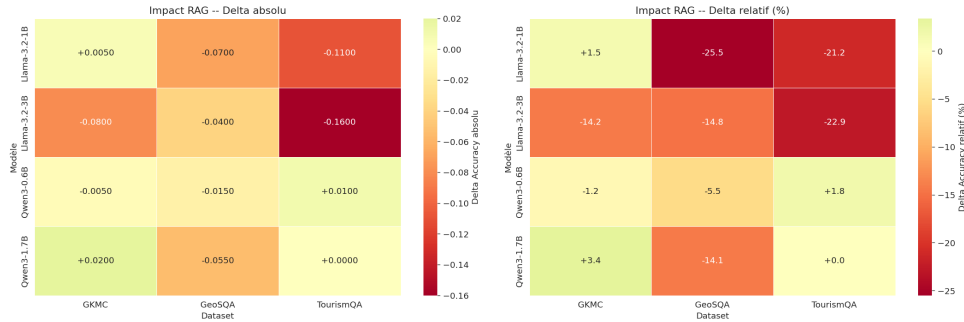
Figure 12 – Heatmap de l'impact du RAG ( \Delta_{rel} ) par modèle et dataset.
