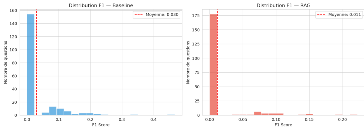
Figure 3 — Distribution des scores F1 par question en mode Baseline (gauche) et RAG (droite). La ligne rouge indique la moyenne.
