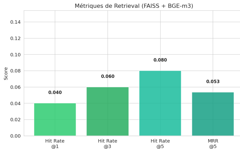
Figure 4 – Métriques de retrieval (Hit Rate@K et MRR@5) sur GeoSQA, étape 1.
