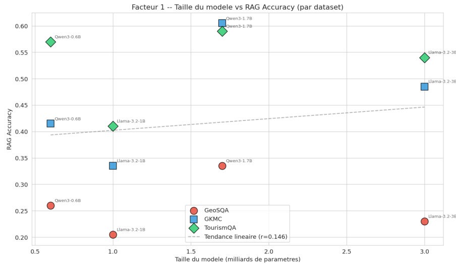
Figure 9 – Relation entre taille du modèle et RAG Accuracy sur les 3 datasets.
