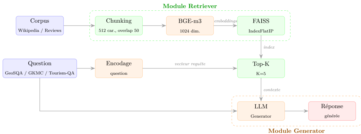
Figure 1 – Architecture du pipeline RAG GeoR2LLMs. Le corpus est découpé en chunks, encodé par BGE-m3 et indexé dans FAISS. Les questions sont encodées, puis les top-K passages récupérés sont fournis comme contexte au générateur LLM.
