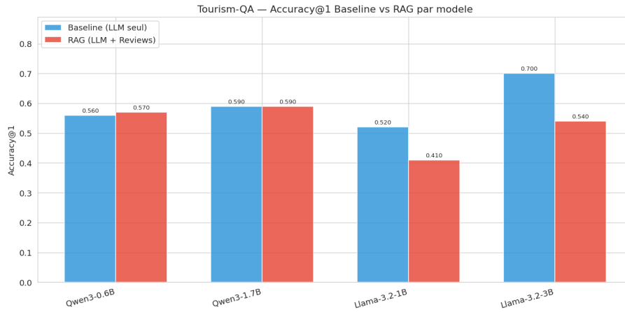
Figure 8 – Accuracy@1 Baseline vs RAG sur Tourism-QA (100 questions, 4 modèles).
