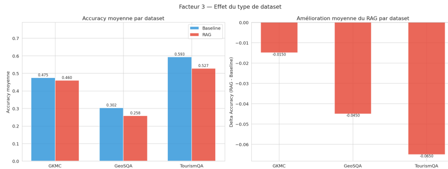
Figure 11 – Difficulté comparée des 3 datasets (RAG Accuracy moyenne).
