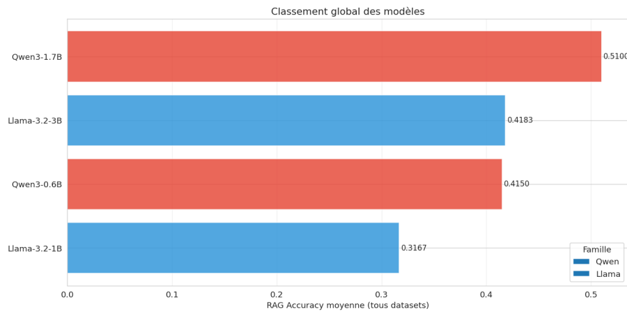
Figure 13 – Classement final des modèles (RAG Accuracy moyenne sur 3 datasets).
