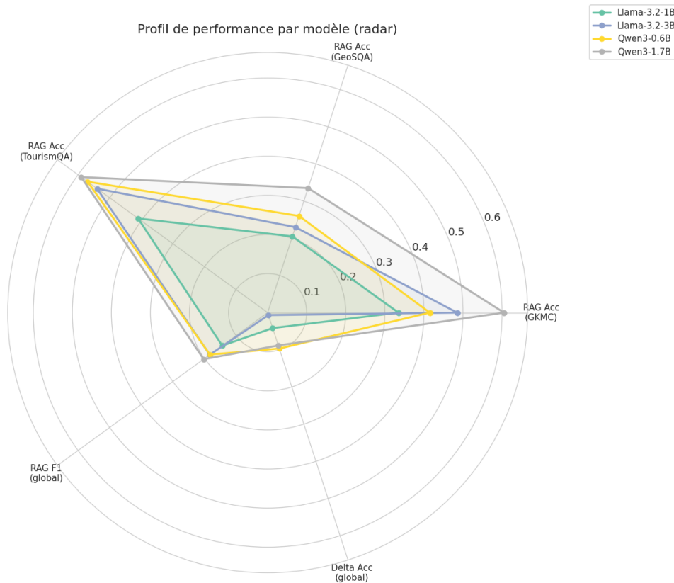
Figure 14 – Profil radar des 4 modèles sur les 3 datasets.
