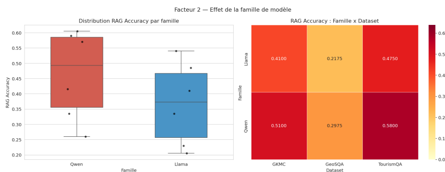
Figure 10 – Analyse comparative des familles Qwen et Llama.
