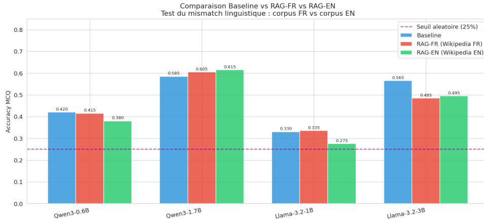
Figure 6 – Comparaison Baseline vs RAG sur GKMC, 4 modèles.
