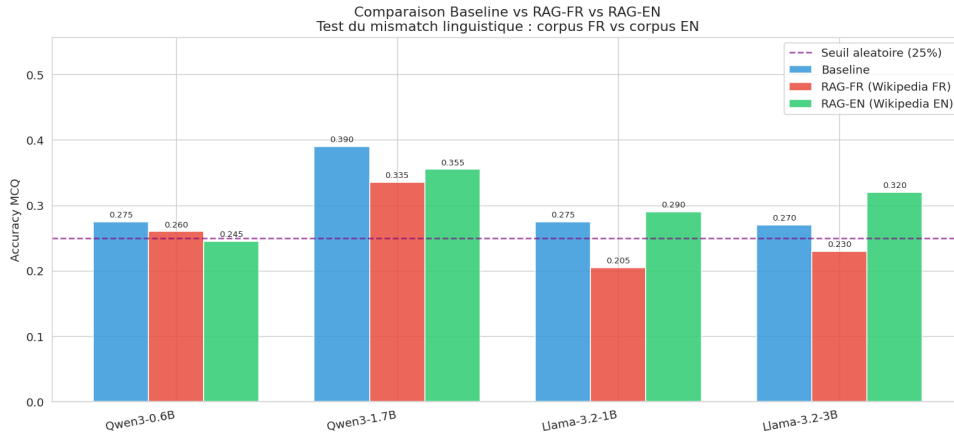
Figure 5 – Comparaison Baseline vs RAG (corpus FR et EN) sur GeoSQA, 4 modèles.
