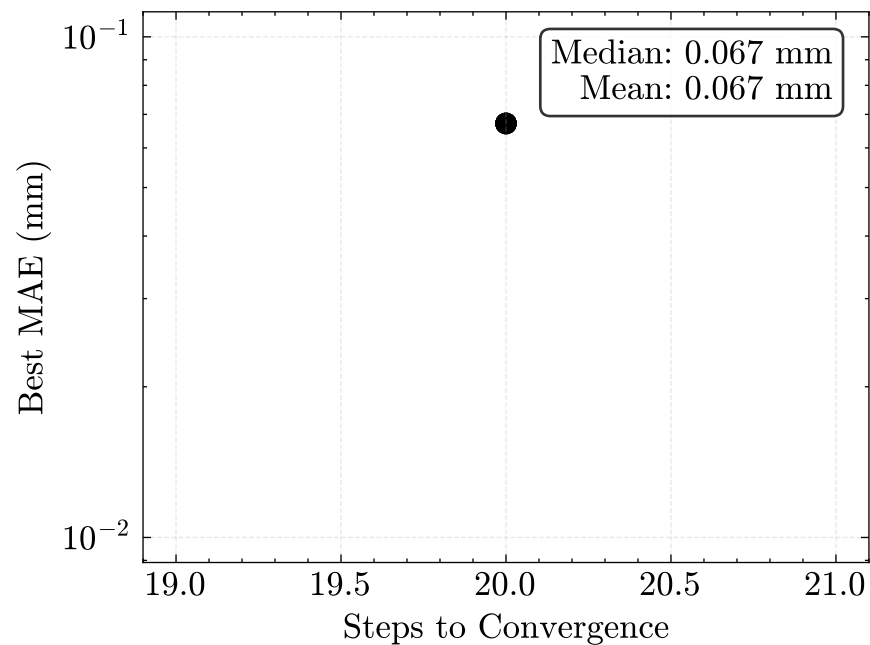
Nelder-Mead
