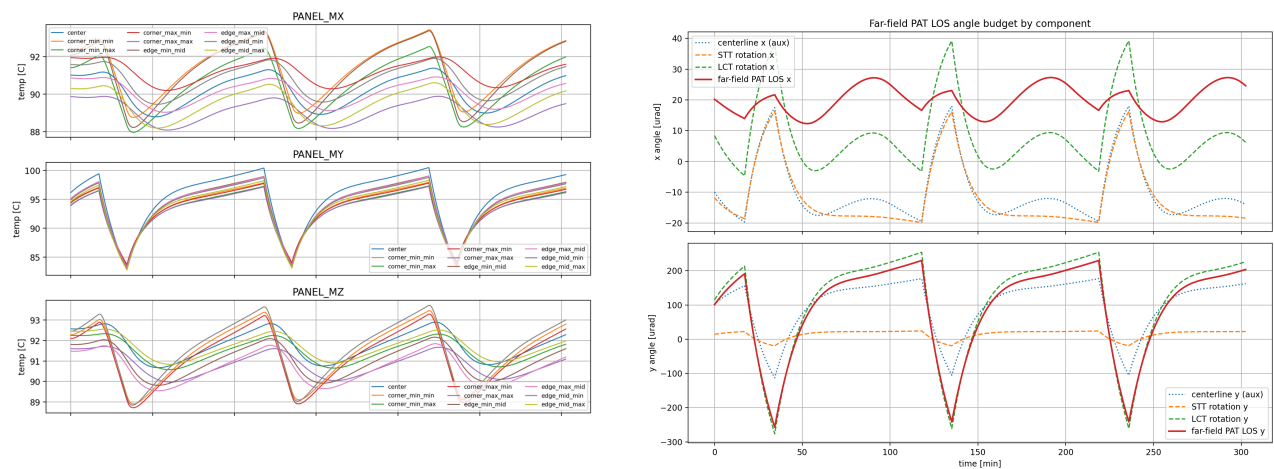
図 4. 代表ケース（Case 04、MY 太陽指向、ALL HEAT）の観察。左: 各パネル代表点の温度時系列。右: STT 相対 LOS
