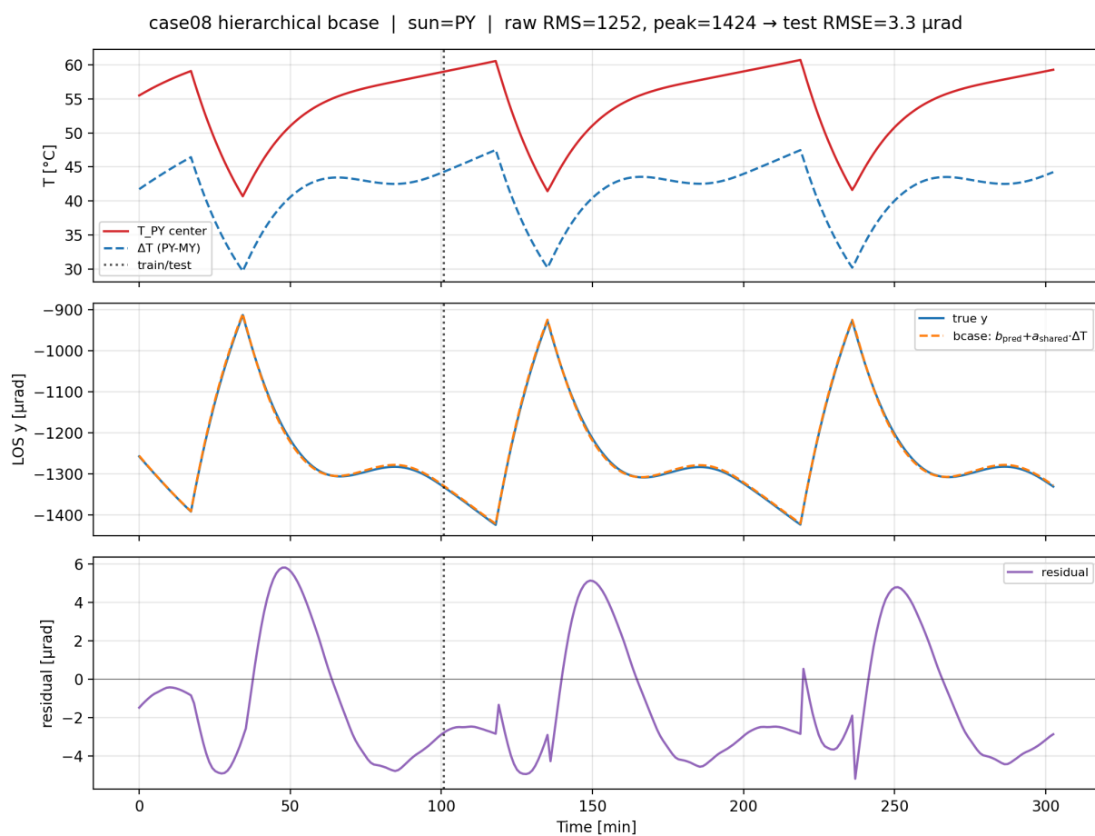
図 7. PY 太陽指向ケースにおける階層モデル予測例。 b_{\text{pred}} + a_{\text{shared}} \Delta T(t) により、大きな軌道内熱 LOS 変動を追従できている。
