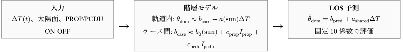
図 5. 階層 sun-face \Delta T モデルの構成。軌道内の時変成分はパネル温度差 \Delta T(t) に割り当て、 \Delta T に入りきらないケース間 DC バイアスを太陽面と内部発熱フラグで説明する。
