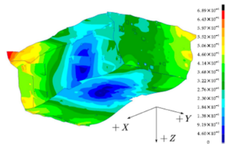
図1 衛星構体の熱変形解析例 3)
