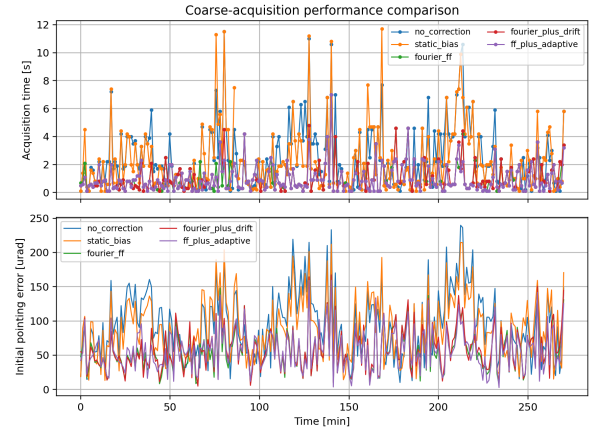
図4 粗捕捉時間と初期指向誤差の比較
