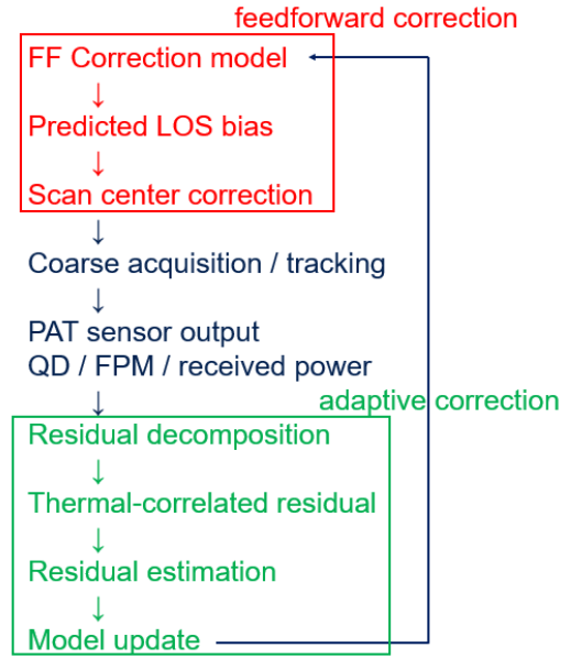
図2 Feedforward 補正と adaptive 補正を組み合わせた二層補正フレームワーク
