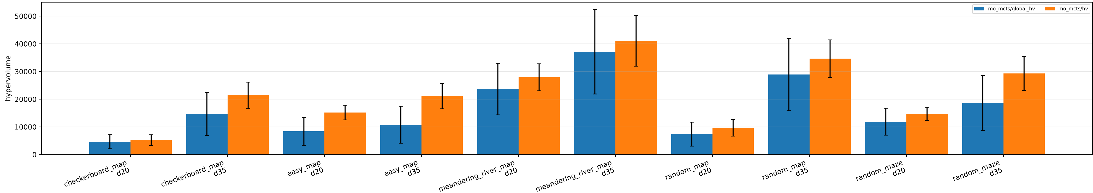
E3 root_selection — HV per (map, dim)
