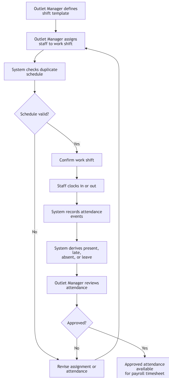
Hình 5: Luồng use case cho phân ca và chấm công
