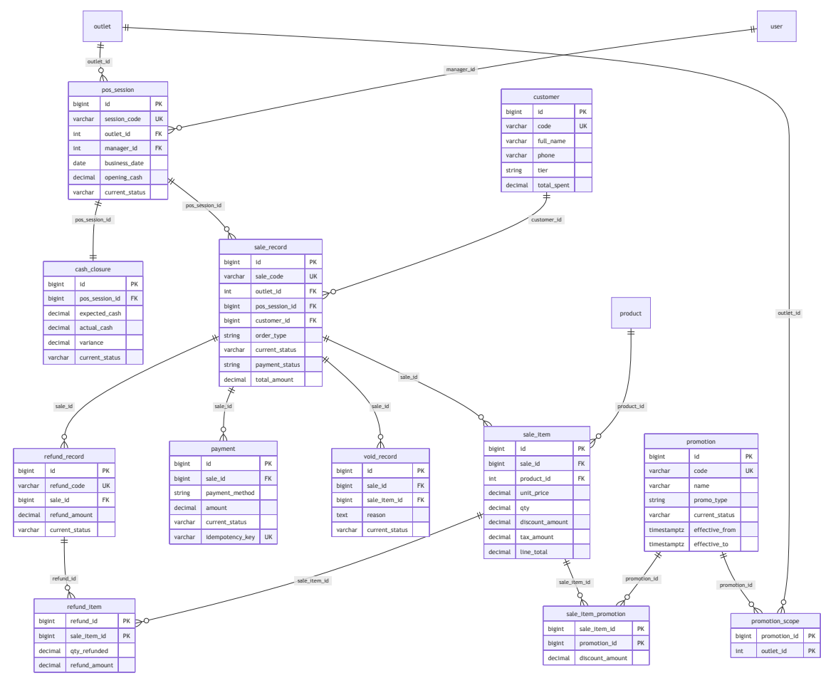
Hình 26: ER Diagram – Sales / POS
