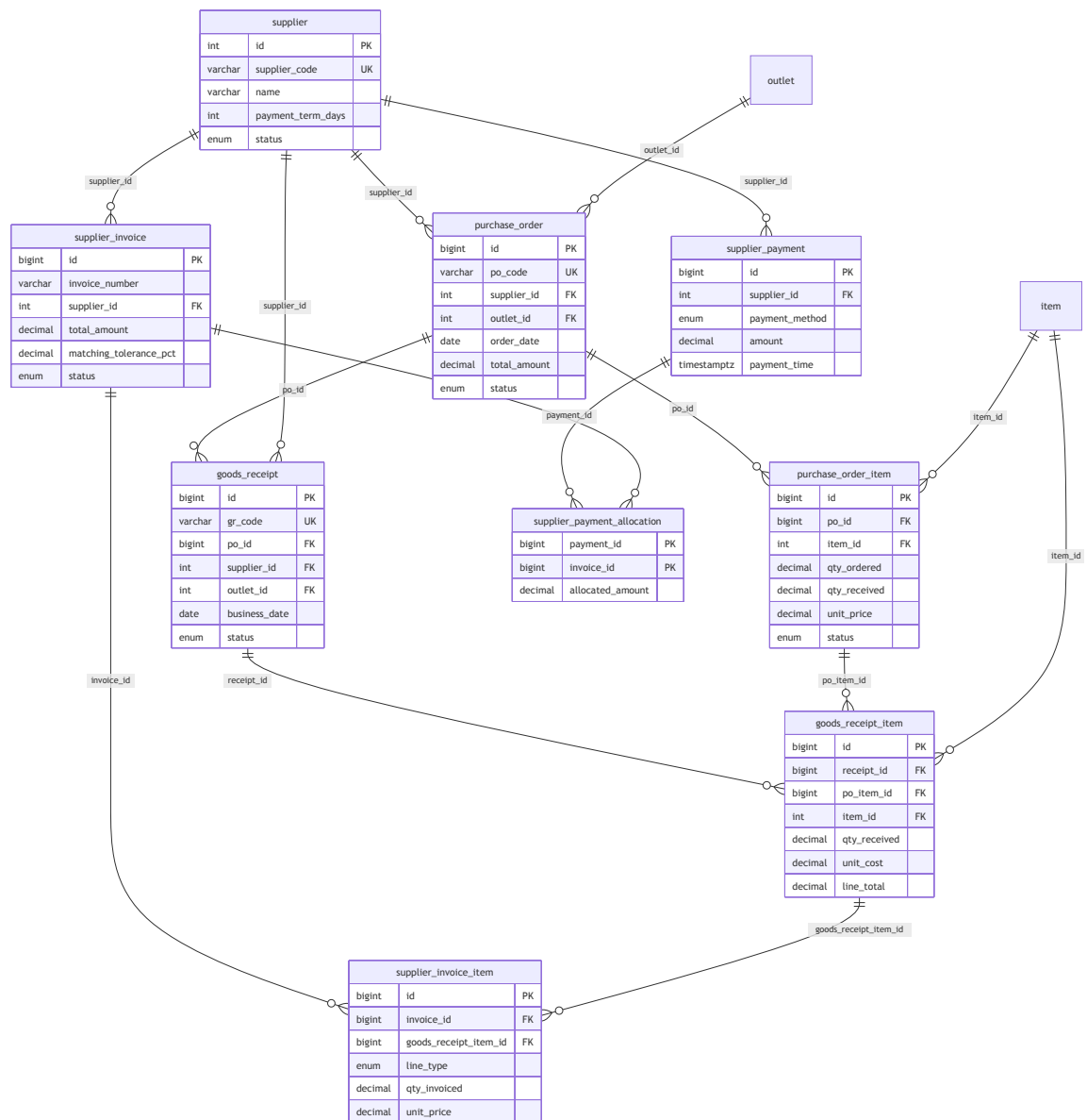
Hình 25: ER Diagram – Procurement (Procure-to-Pay)
