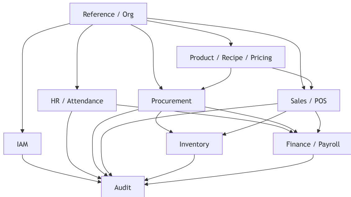
Hình 1: Sơ đồ tương tác module cấp cao
