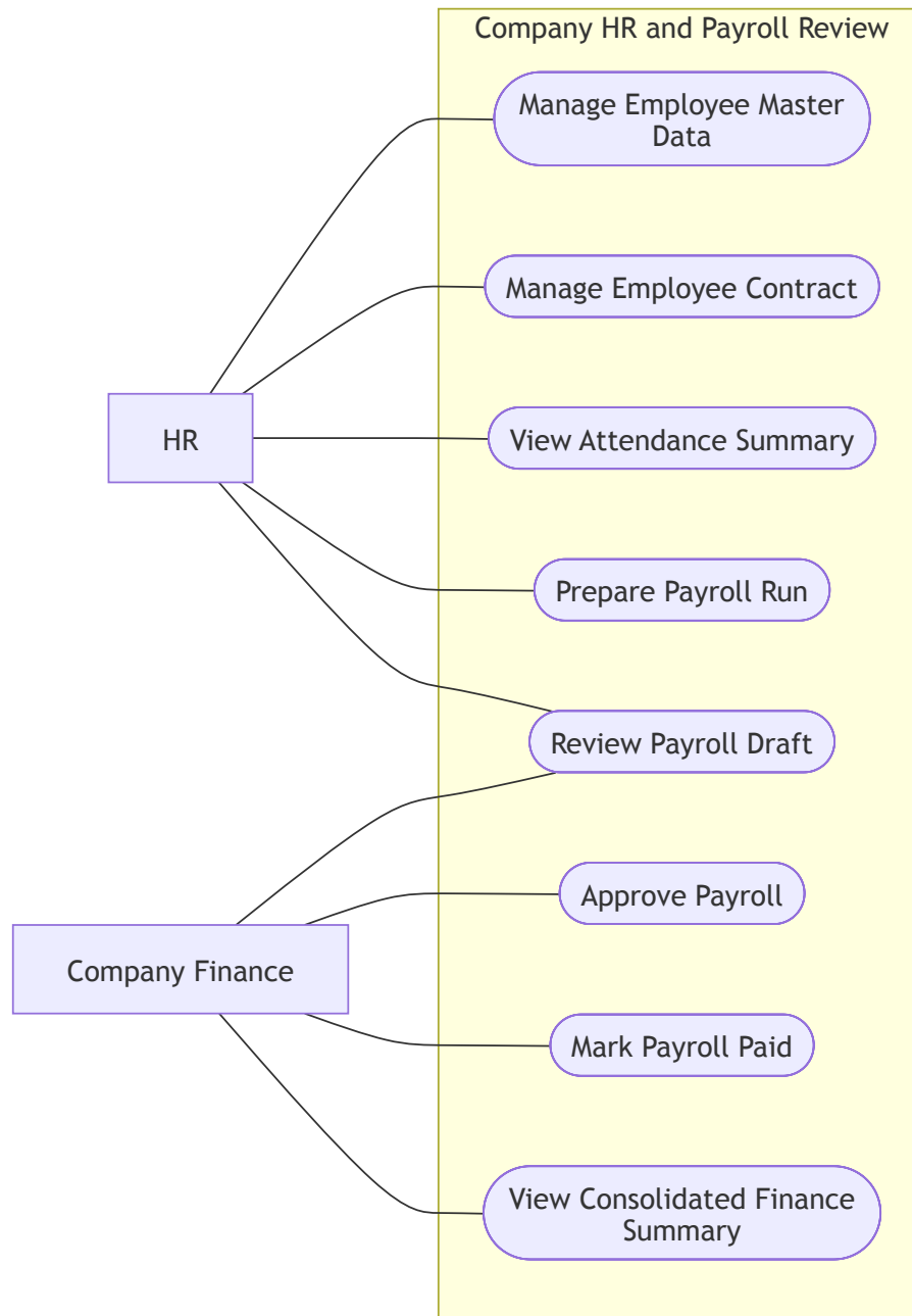
Hình 20: Biểu đồ 09: HR và payroll ở cấp hệ thống
