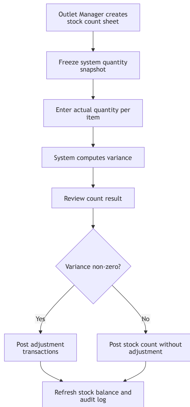
Hình 9: Luồng use case cho stock count và inventory adjustment
