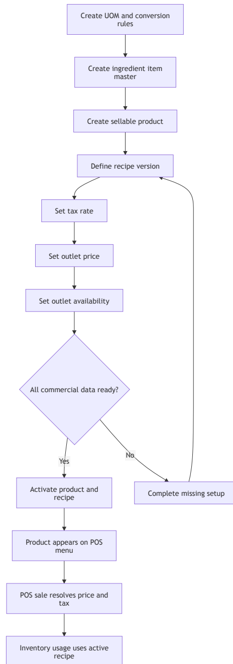
Hình 6: Luồng use case cho sản phẩm, công thức và định giá
