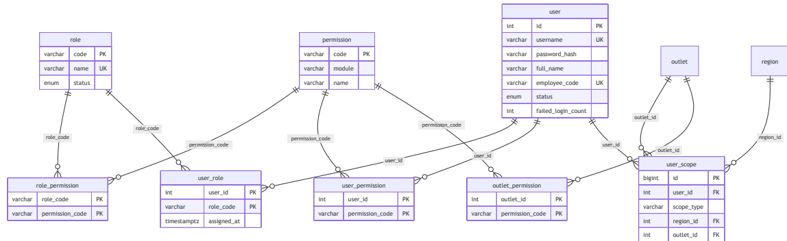
Hình 22: ER Diagram – Identity & Access Management
