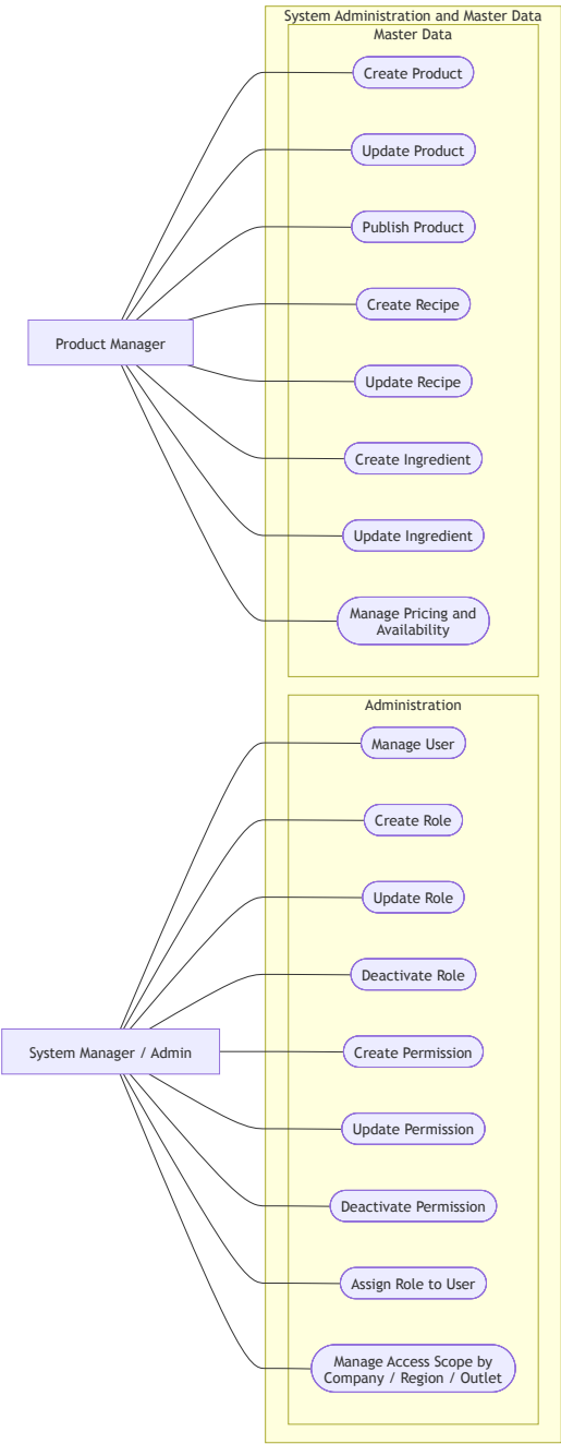
Hình 19: Biểu đồ 10: Quản trị hệ thống và dữ liệu chủ
