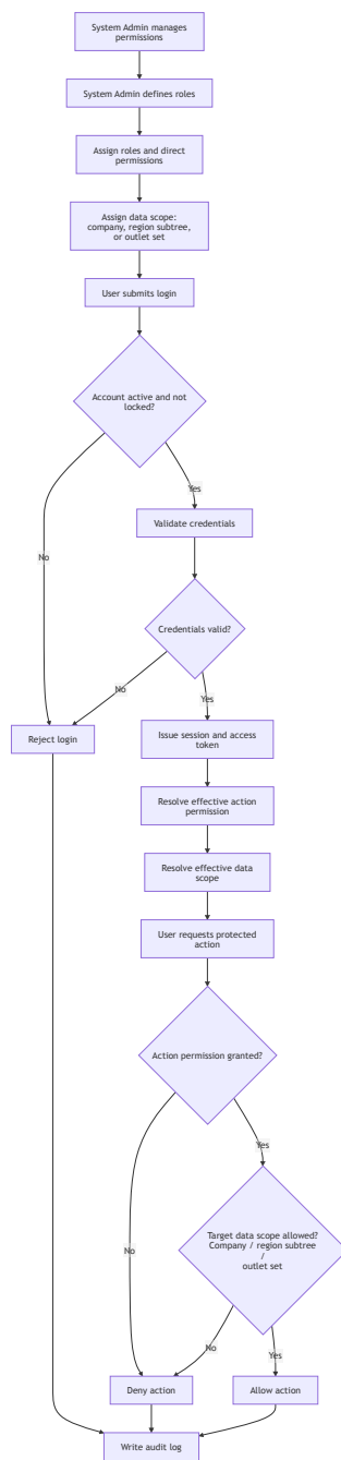
Hình 4: Luồng use case cho IAM và phân quyền
