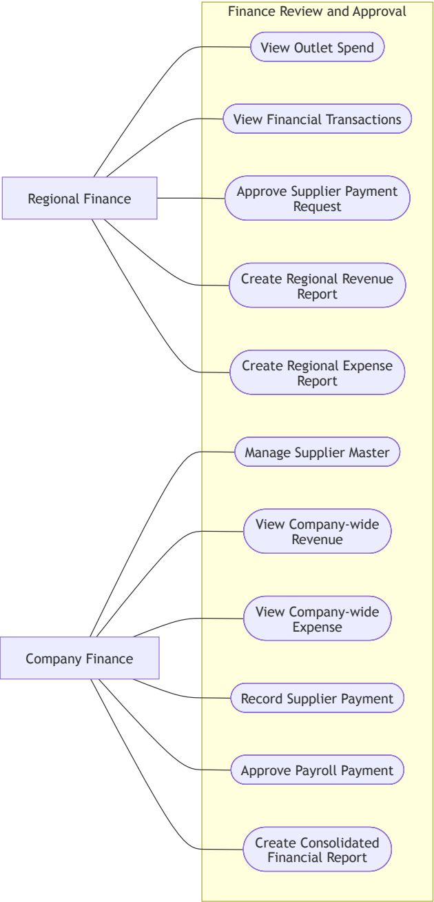
Hình 16: Biểu đồ 06: Tài chính vùng, tài chính công ty và supplier master
