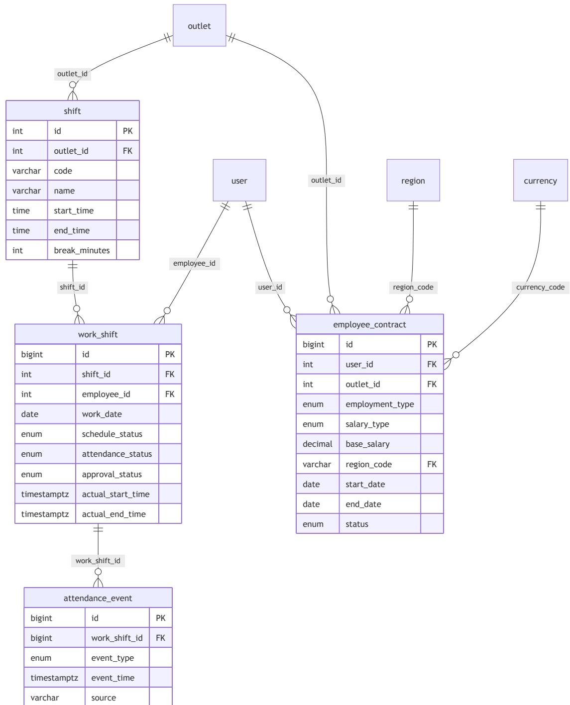
Hình 23: ER Diagram – HR & Attendance
