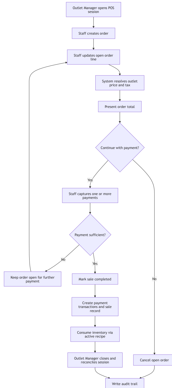
Hình 8: Luồng use case cho bán hàng và vận hành POS
