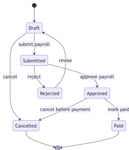
Hình 2: State machine cho payroll
