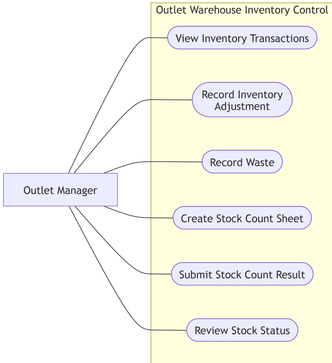
Hình 15: Biểu đồ 05: Kiểm soát tồn kho tại outlet
