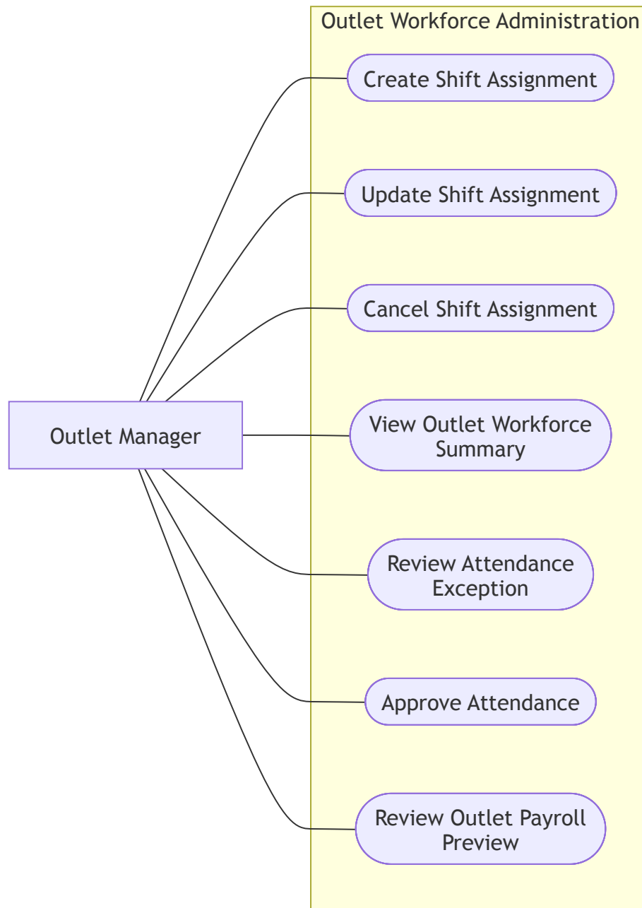
Hình 18: Biểu đồ 08: Vận hành lực lượng lao động tại outlet
