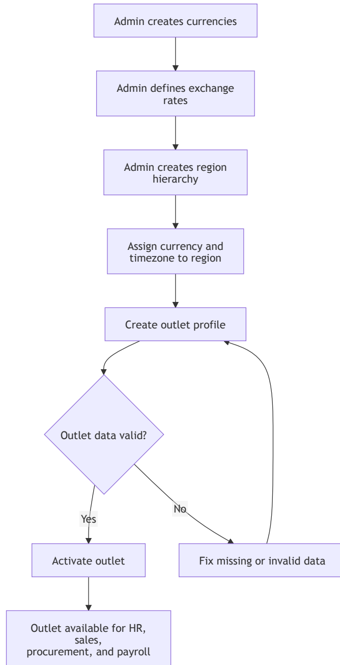
Hình 3: Luồng use case cho thiết lập tham chiếu và tổ chức
