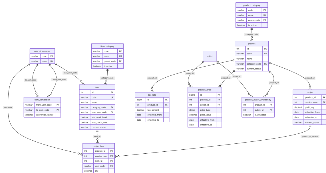
Hình 24: ER Diagram – Product, Recipe & Pricing
