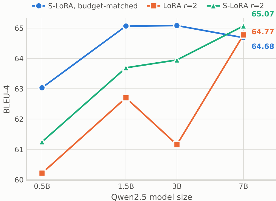
E2E NLG, bfloat16
