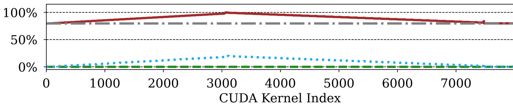
(d) Granite-3B-Instruct BS=2
