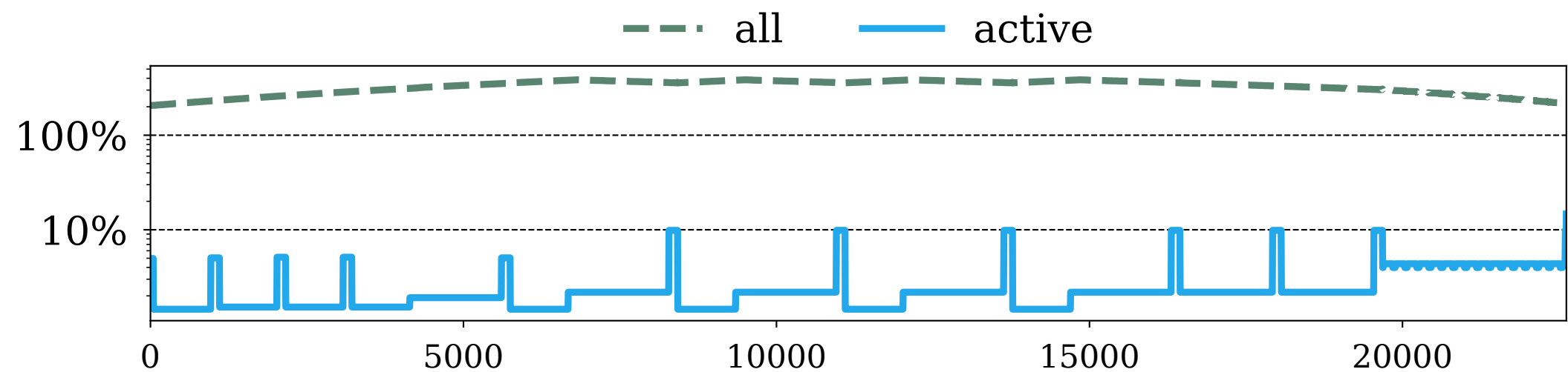
(d) GPT2-40B-GPU0
