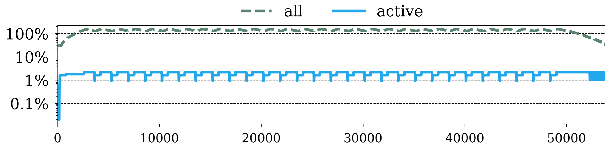
(a) Llama3-8B-GPU0
