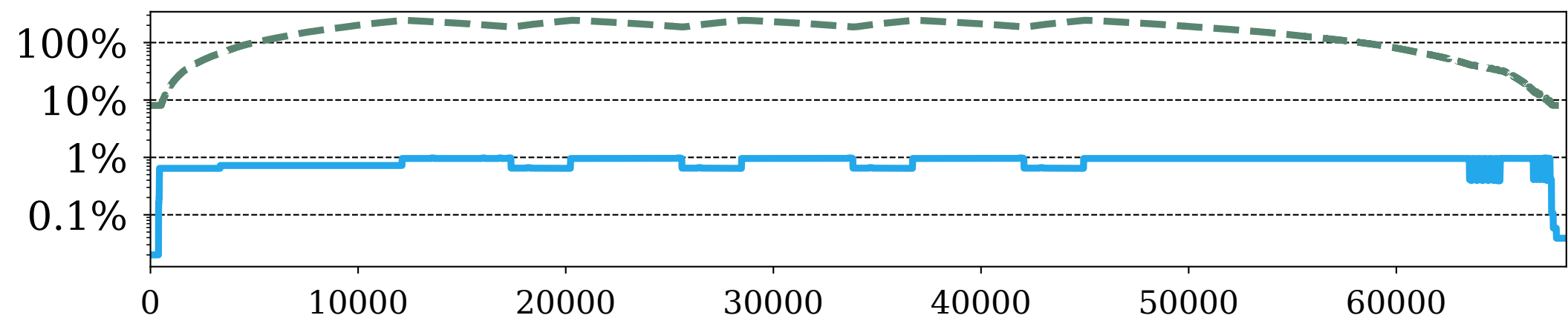
(d) GPT2-40B-GPU0
