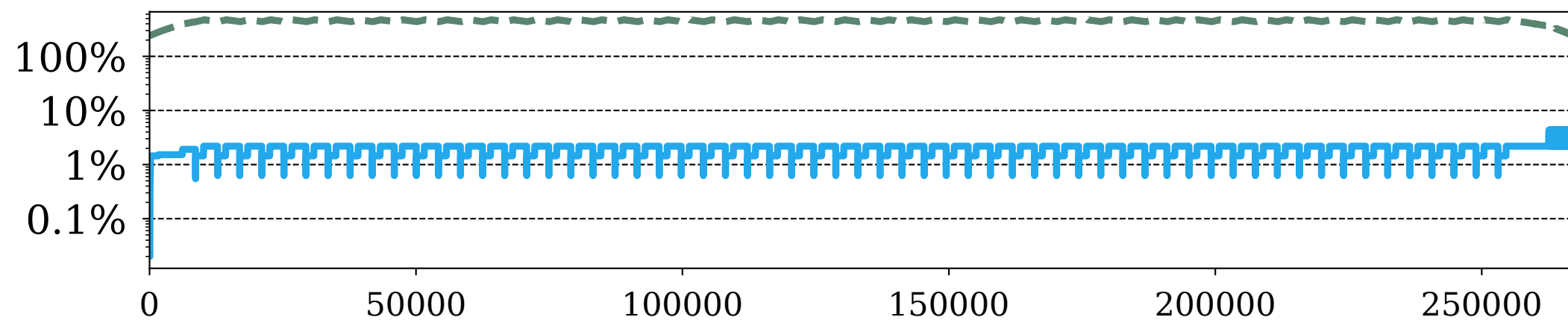
(a) Llama3-8B-GPU0
